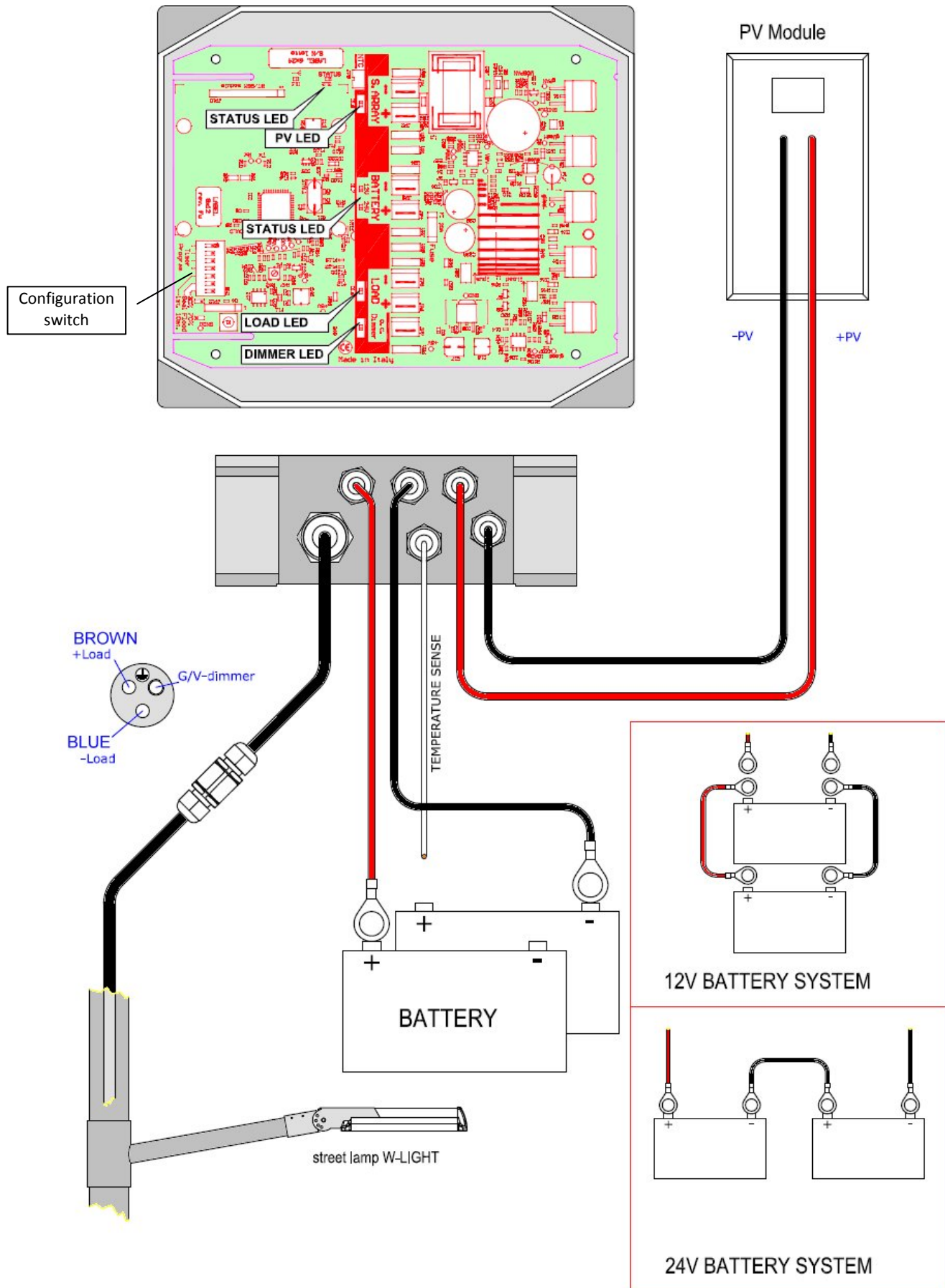
Fig. 1 Wiring scheme
