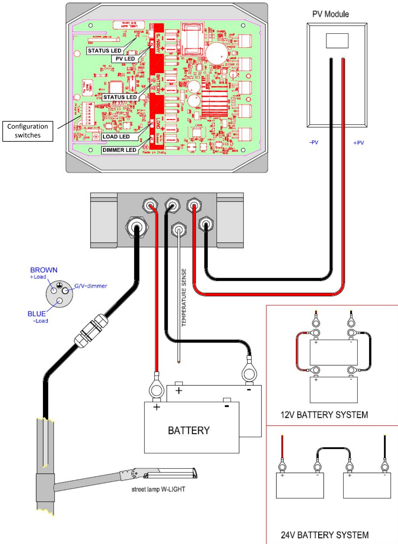
Fig. 1 Schema di cablaggio
